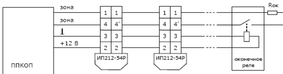
Рисунок 6 - Схема подключение извещателей ИП212-54Р к ПКПОП с использованием оконечного реле для контроля наличия напряжения питания.
