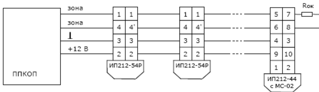
Рисунок 5 - Схема подключение извещателей ИП212-54Р к ПКПОП с использованием ИП212-44 с МС-02 для контроля наличия напряжения питания.
