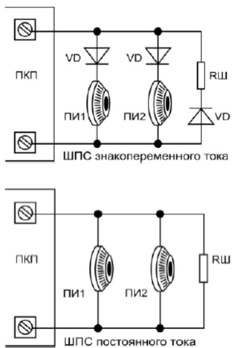
Рис.1. Типовые схемы подключения. Рис.2. Схемы подключения извещателя к ШС.
