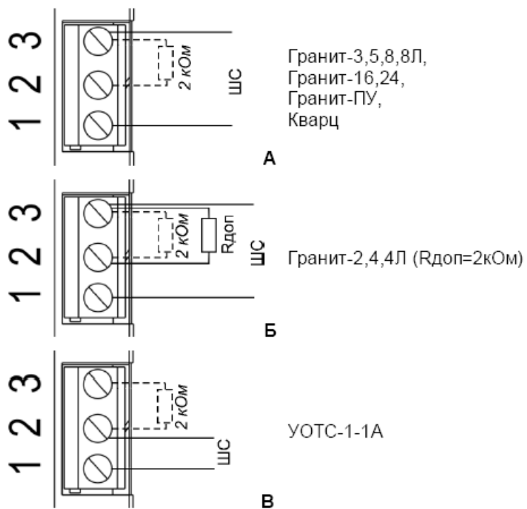
Рис.1. Типовые схемы подключения. Рис.2. Схемы подключения извещателя к ШС.
