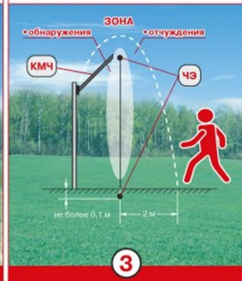
ВАРИАНТЫ УСТАНОВКИ ЧУВСТВИТЕЛЬНЫХ ЭЛЕМЕНТОВ (ЧЭ)
