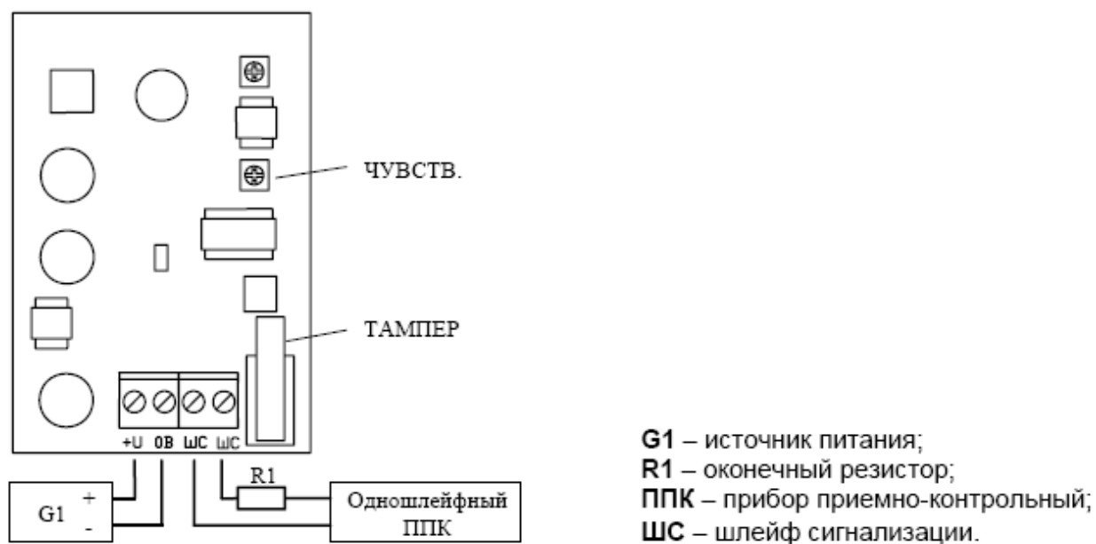
Рисунок 1 Схема подключения извещателя
