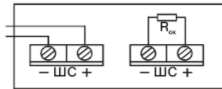
б) при включении на конце ШС
